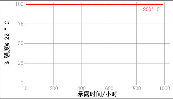
热老化曲线 在所示温度下老化，测试温度是22 ° C
