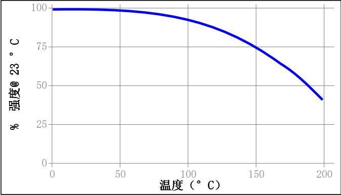
热老化 在所示温度下老化, 测试温度为23° C
