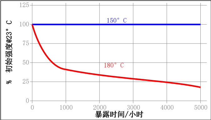
耐化学品/溶剂性能 在下列条件下进行老化, 然后在23° C下测试
